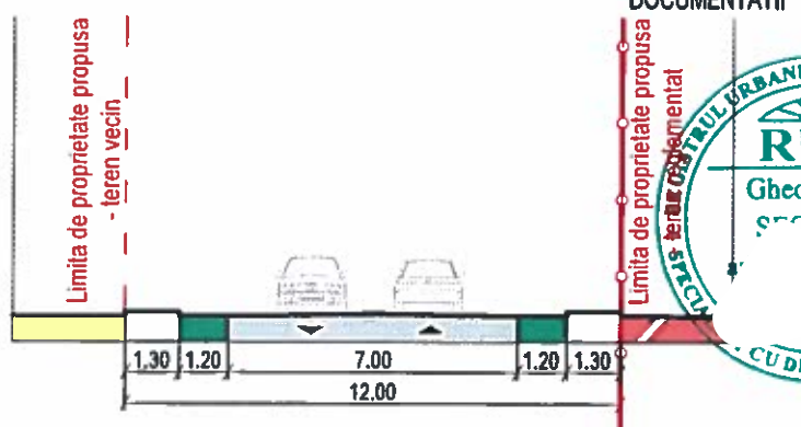
SECTIUNE PROFIL STRADAL PROPUS
